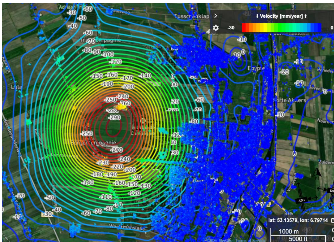
Figuur 4.3 Bodemdalingcontouren Insar feb 2016 t/m juni 2026 in mm. De gekleurde punten geven de gemiddelde dalingsnelheid van meetpunten van 0 tot 30 mm/jaar. De contouren hebben hun eigen kleurenschaal van 0 tot 290 mm.
