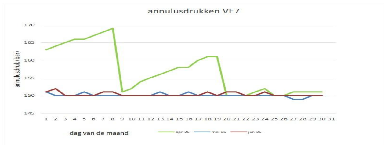
Figuur 1.7 Drukken VE-7 afgelopen kwartaal
