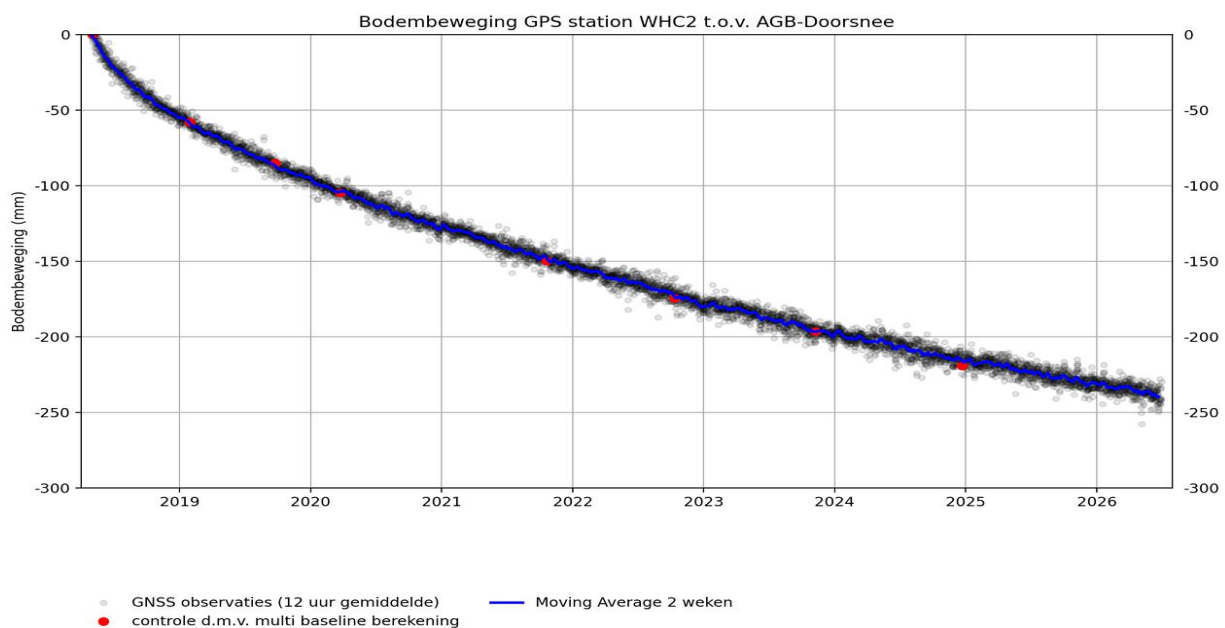
Figuur 4.2 GPS dagwaardes en 14-daagse gemiddelde voor bodemdaling op WHC-2 sinds mei 2018. De spreiding is meetruis (meteorologische effecten), die over een langere periode uitmiddelt.
