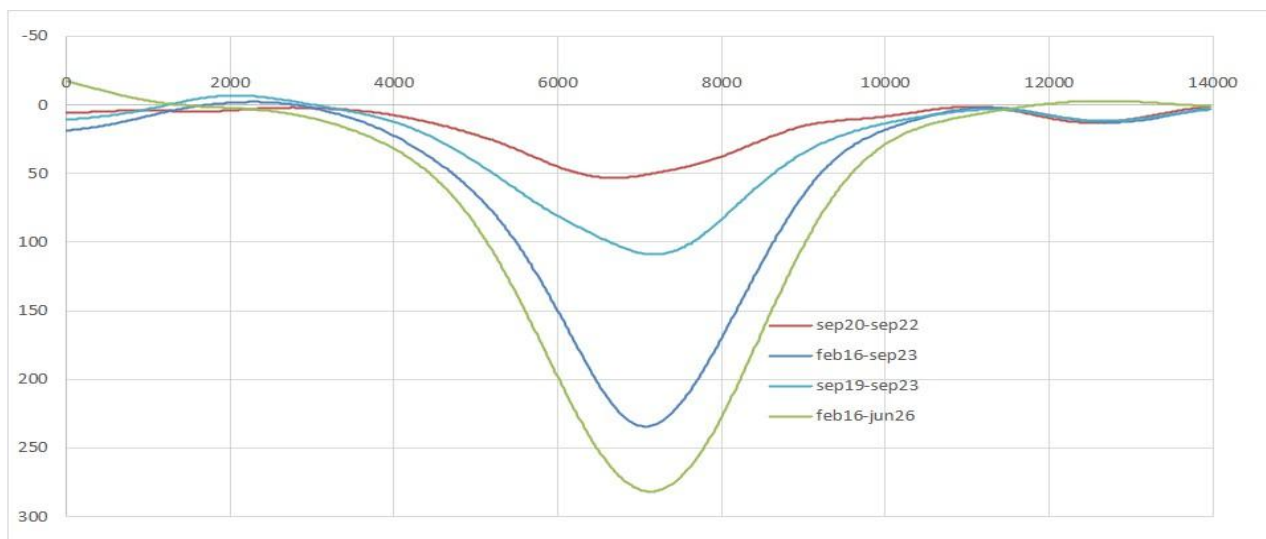
Figuur 4.6 : Insar bodemdaling W-E feb 2016 – juni 2026 en drie andere periodes.
