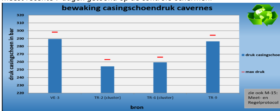
Figuur 1.2 Screenshot als voorbeeld (dec 2025) van drukken en maximum drukken op casingschoenniveau voor het cluster (putten TR-2 en back-up meting TR-6) en voor de cavernes VE-3 en TR-9.
