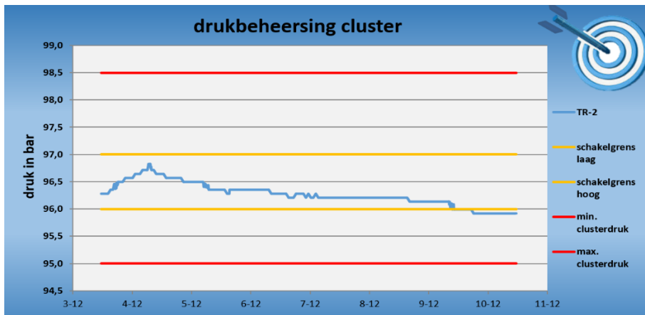
Figuur 1.1 Screenshot als voorbeeld (dec 2025) van de drukbeheersing cluster, basis TR-2 Het drukverloop van TR-2 over het afgelopen kwartaal staat in Fig 1.3. In de controlekamer worden de meest recente 7 dagen getoond op de controle-schermen.
