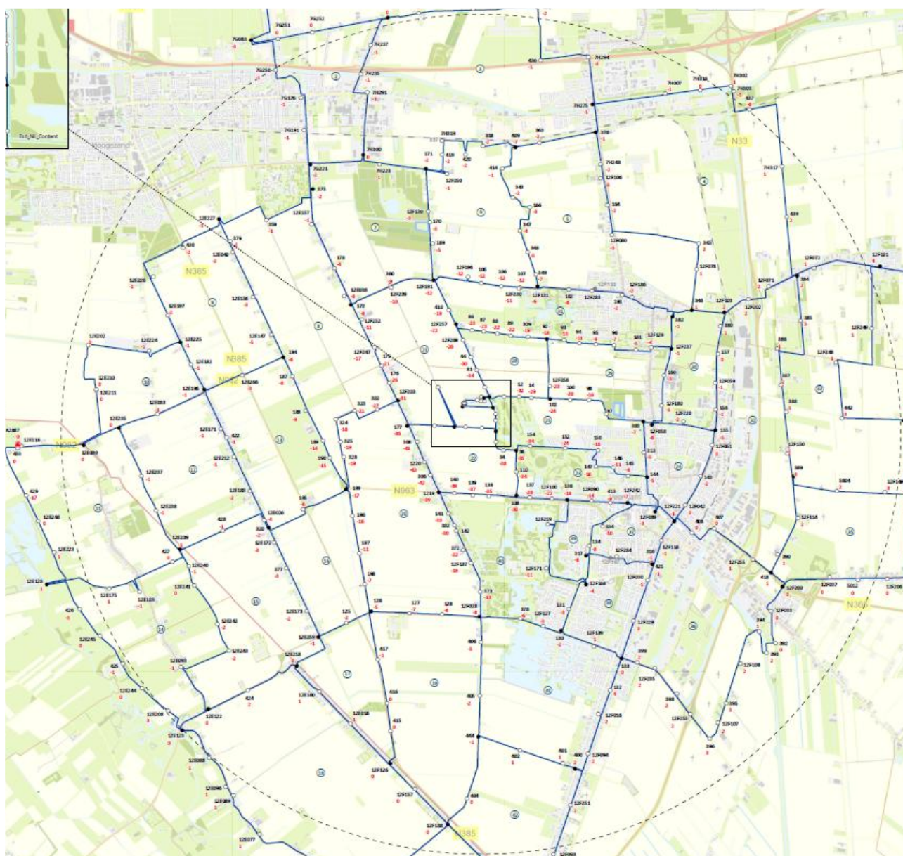
Figuur 4.4: Waterpasmeetnet Nedmag in 2024, deels overlappend met het NAM meetnet met dalingen (indien negatief) in mm tussen 2022 en 2024.
