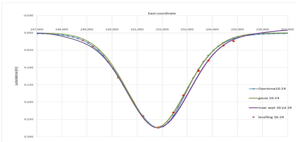
Figuur 4.7 : fit west-oost bodemdaling volgens Geertsma (SGS-model), Gauss curve, Insar en waterpas (levelling) data 2016-2024, als functie breedte-coordinaten (Easting). Northing is 571 088 m.
