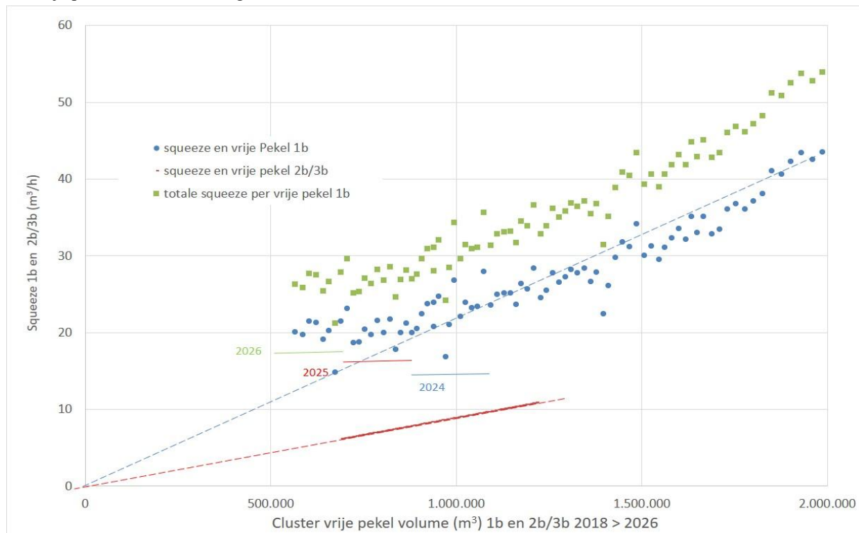
Fig A.1 Convergentiesnelheid van TR-cluster bij bijna constante cavedruk als functie van het geschatte vrije volume van de 1b (bischofiet) sectie en de 2b/3b carnallietsectie. Aan de rechterzijde is eind 2019 met 55 m 3 /h convergentie en de linkerzijde het afgelopen kwartaal met circa 25 m 3 /h. De meeste convergentie komt uit de bischofiet-sectie, waar aangenomen wordt dat de carnallietsectie langzamer convergeert met circa 8 m 3 /h.
