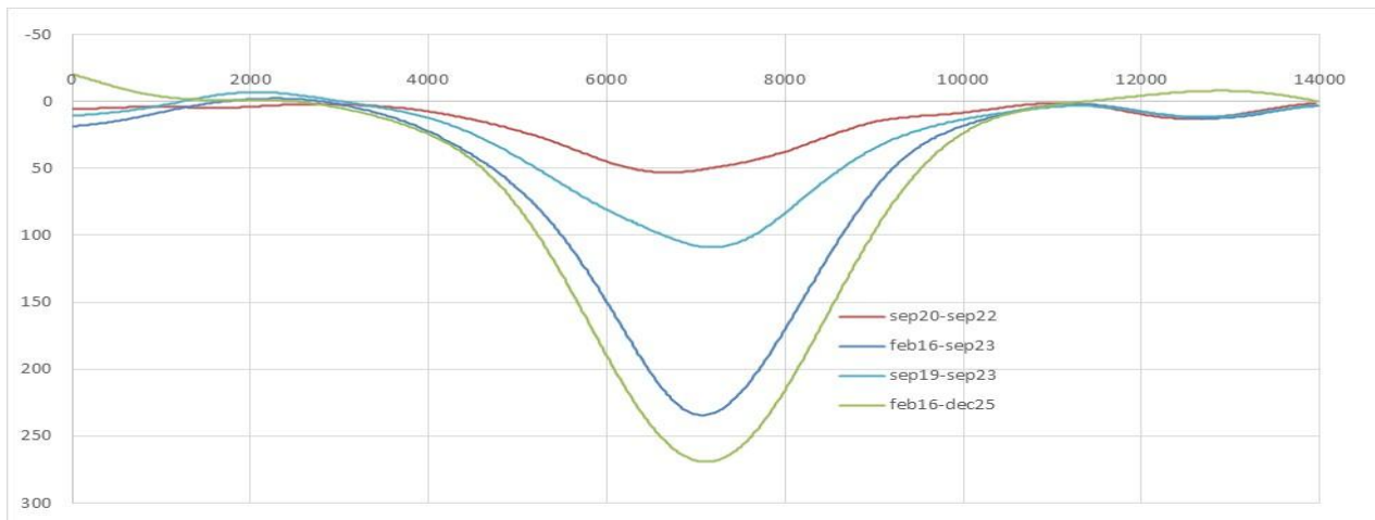
Figuur 4.6 : Insar bodemdaling W-E feb 2016 – dec 2025 en drie andere periodes.
