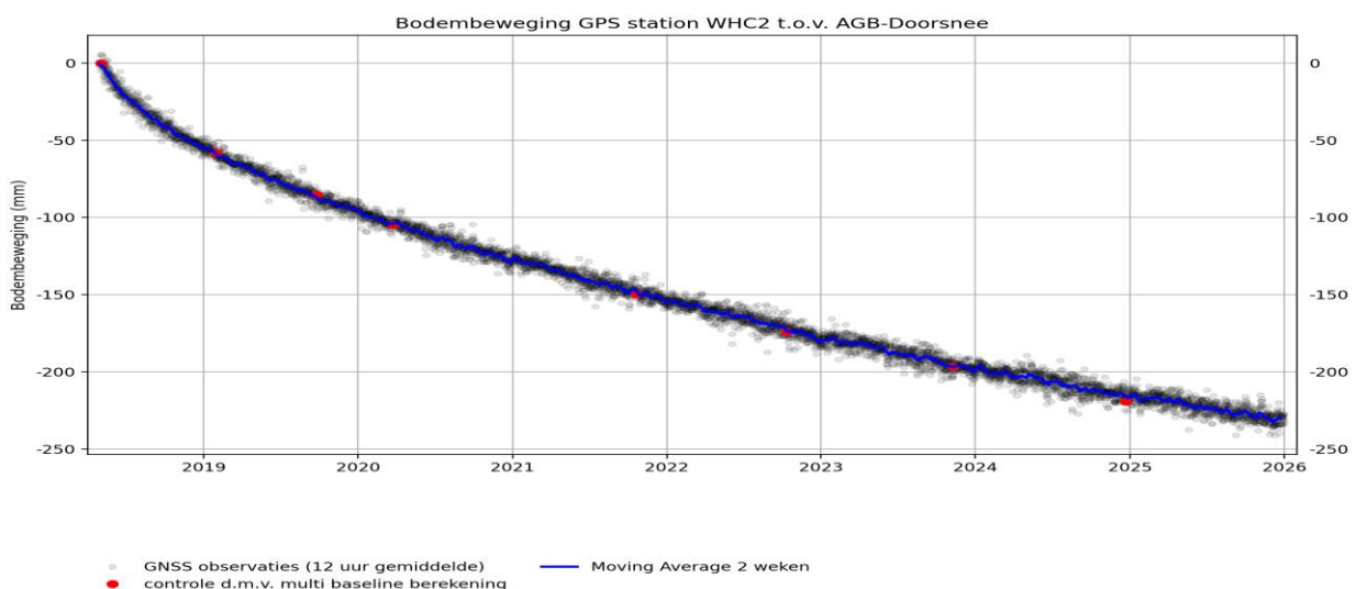
Figuur 4.2 GPS dagwaardes en 14 daagse gemiddelde voor bodemdaling op WHC-2 sinds mei 2018. De spreiding is meetruis (meteorologische effecten), die over een langere periode uitmiddelt.
