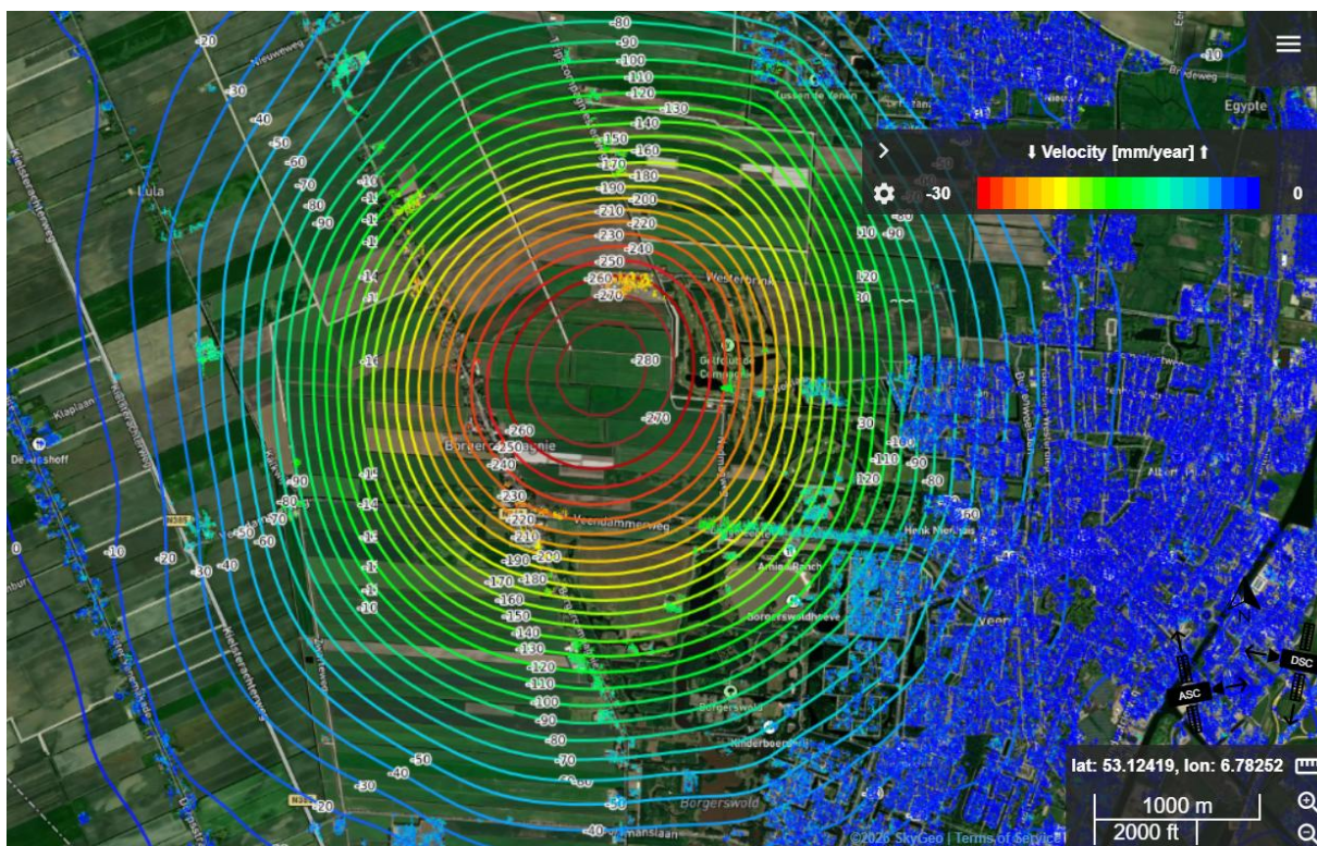
Figuur 4.3 Bodemdalingcontouren InSar feb 2016 t/m dec 2025 in mm. De gekleurde punten geven de gemiddelde dalingsnelheid van meetpunten van 0 tot 30 mm/jaar. De contouren hebben hun eigen kleurschaal van 0 tot 280 mm.
