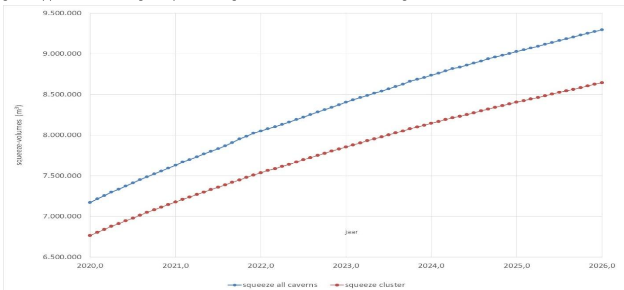
Figuur 4.1: cumulatieve squeeze-evolutie (caverneconvergentie) in m 3 vanaf jan-2020 .
