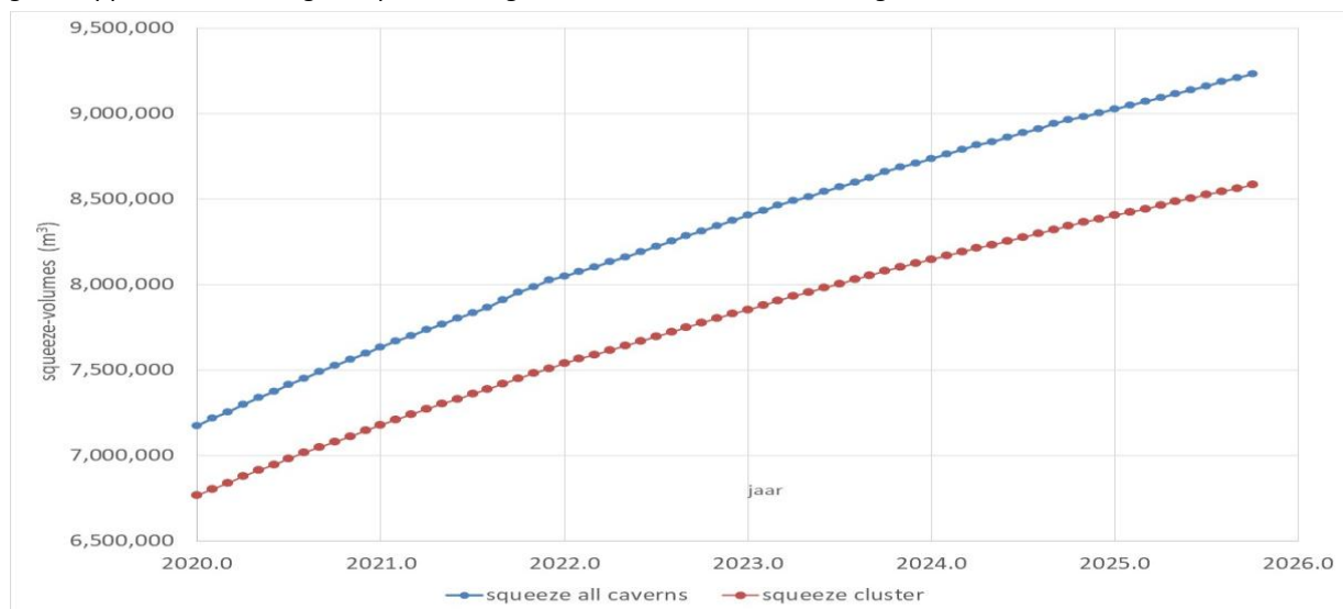
Figuur 4.1: cumulatieve squeeze-evolutie (caverneconvergentie) in m^3 vanaf jan-2020.
