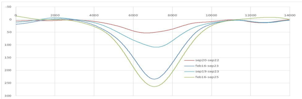
Figuur 4.6 : Insar bodemdaling W-E feb 2016 – sep 2025 en drie andere periodes.
