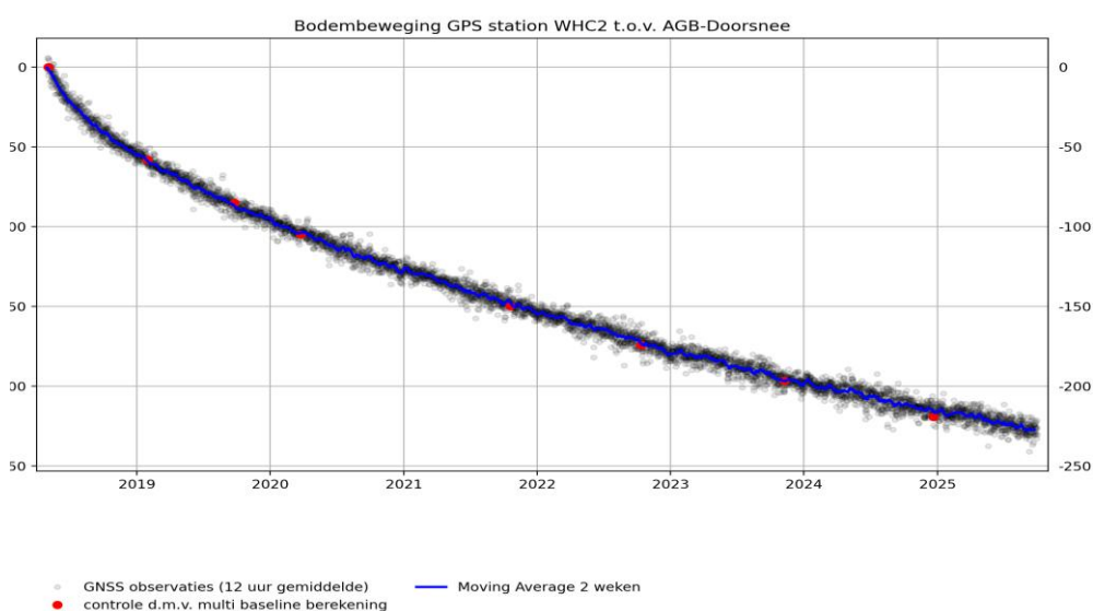
Figuur 4.2 GPS dagwaardes en 14 daagse gemiddelde voor bodemdaling op WHC-2 sinds mei 2018. De spreiding is meetruis (meteorologische effecten), die over een langere periode uitmiddelt.
