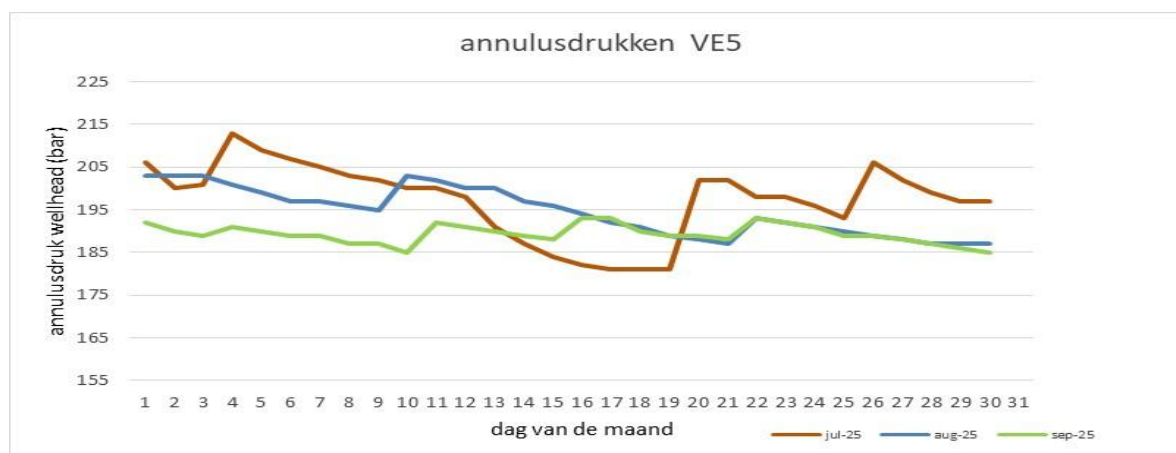
Figuur 5.1 Drukken annulus VE-5.
