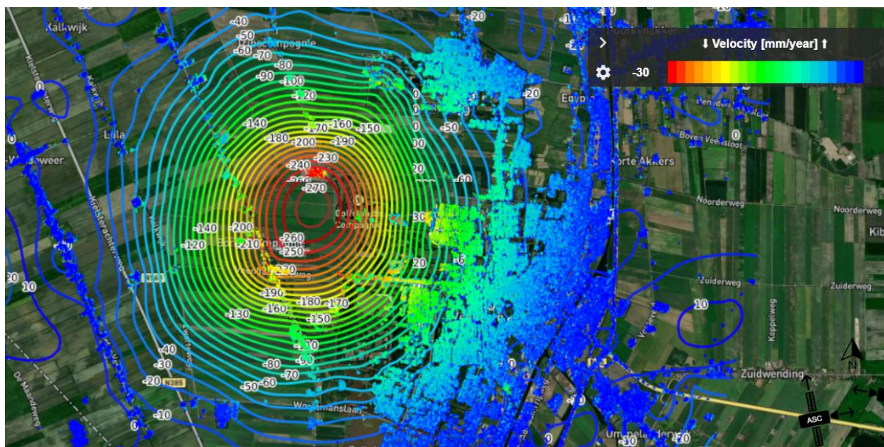
Figuur 4.3 Bodemdalingcontouren Insar feb 2016 t/m sep 2025 in mm. De gekleurde punten geven de gemiddelde dalingsnelheid van meetpunten van 0 tot 30 mm/jaar. De contouren hebben hun eigen kleurenschaal van 0 tot 270 mm.
