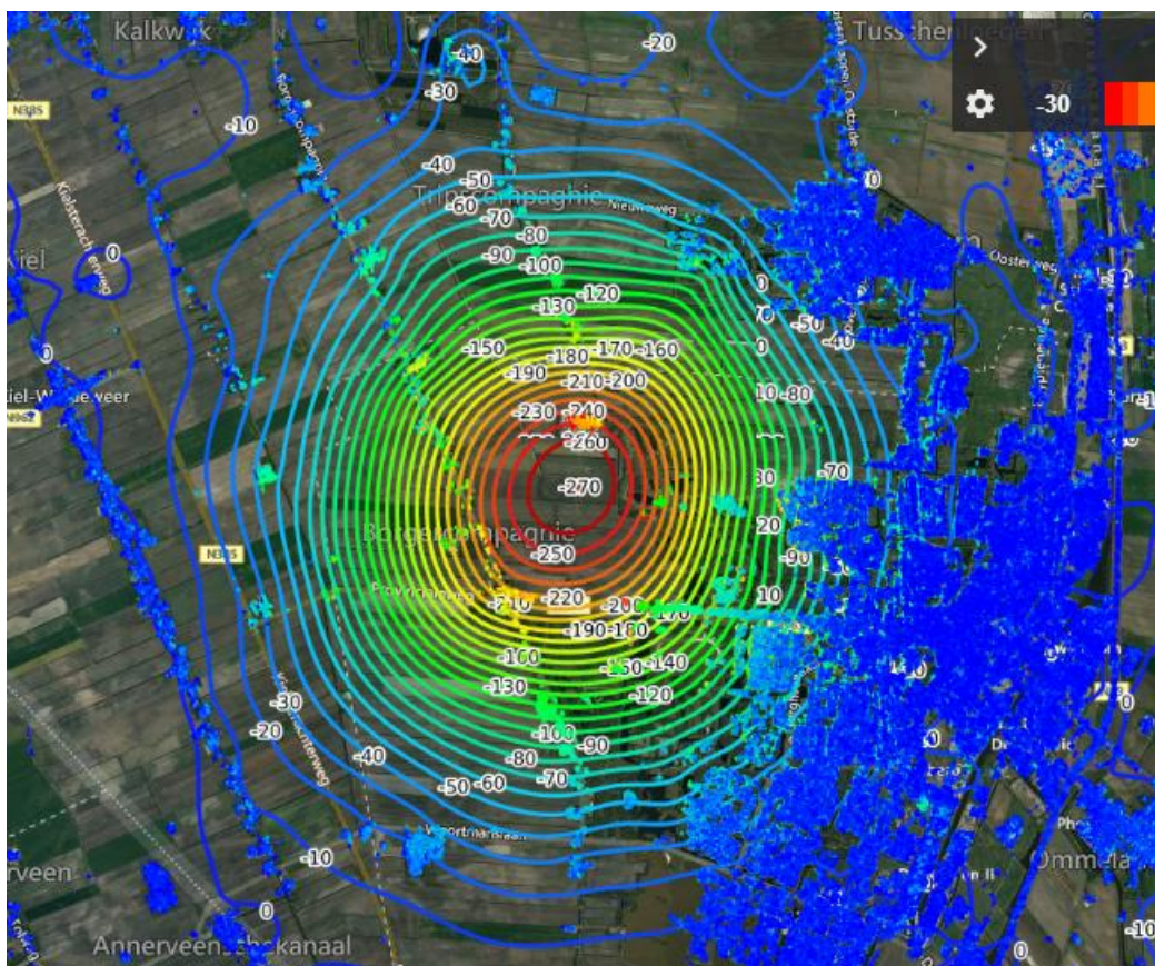
Figuur 4.3 Bodemdalingcontouren Insar feb 2016 t/m mrt 2025 in mm. De gekleurde punten geven de gemiddelde dalingsnelheid van meetpunten van 0 tot 30 mm/jaar. De contouren hebben hun eigen kleurschaal van 0 tot 270 mm.
