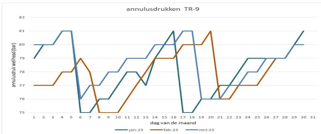
Figuur 1.5 drukverloop annulusdruk van TR-9 in voorgaand kwartaal.
