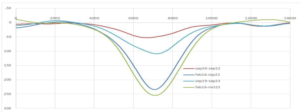
Figuur 4.6 : Insar bodemdaling W-E feb 2016 – maart 2025 en drie andere periodes.
