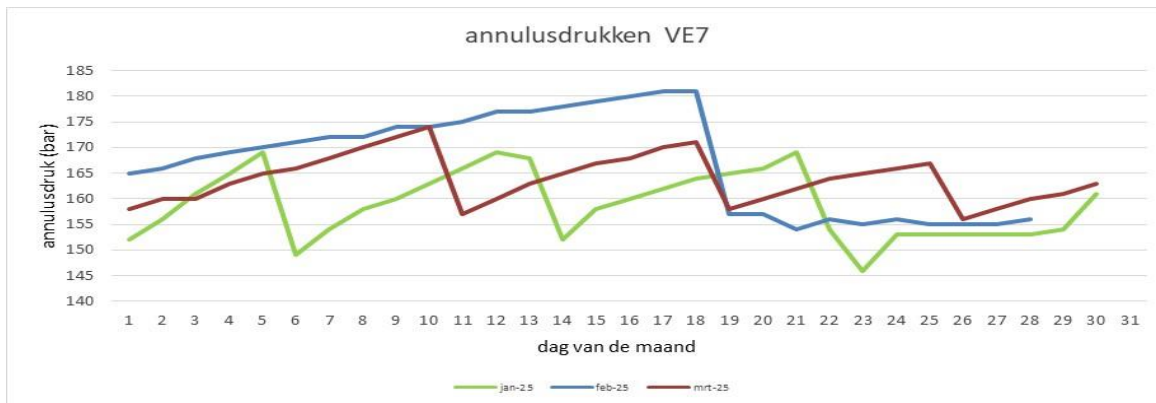
Figuur 5.2 Drukken annulus VE-7. Langzaam oplopende waarden zijn oplos-expansie en kruip.
