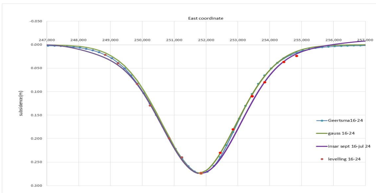
Figuur 4.7 : fit west-oost bodemdaling volgens Geertsma (SGS-model), Gauss curve, Insar en waterpas (levelling) data 2016-2024, als functie breedte-coordinaten (Easting). Northing is 571 088 m.
