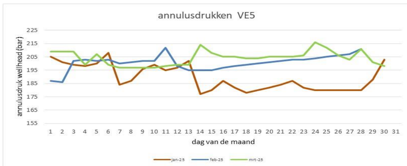
Figuur 5.1 Drukken annulus VE-5.
