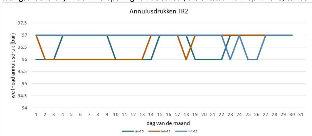
Figuur 1.3 drukverloop TR-2 in voorgaand kwartaal (drukken zijn afgerond op hele bars).
