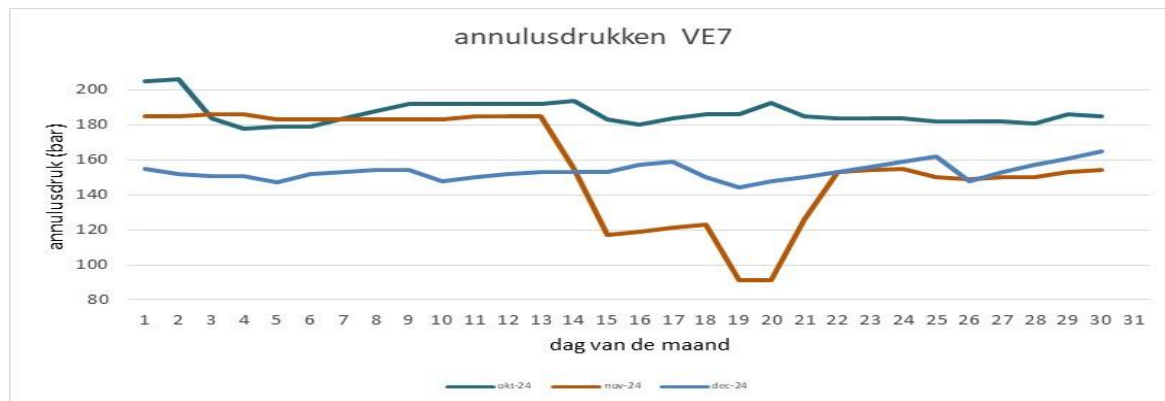
Figuur 5.2 Drukken annulus VE-7. Langzaam oplopende waarden zijn oplos-expansie en kruip. Midden november is de lichte dakolie uit de annulus vervangen door zwaarder water over een periode van circa 1 week, waardoor de wellhead annulusdruk met circa 36 bar vermindert bij gelijke cavernedruk.
