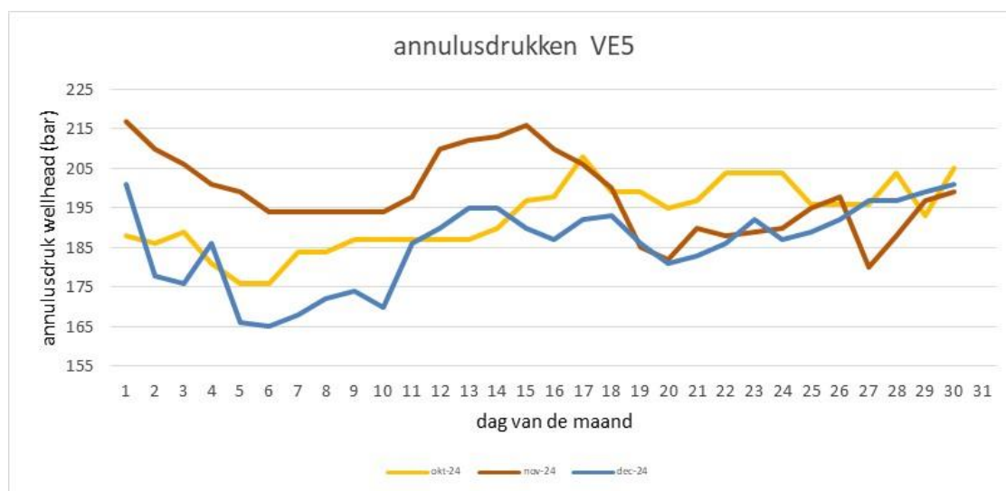
Figuur 5.1 Drukken annulus VE-5.
