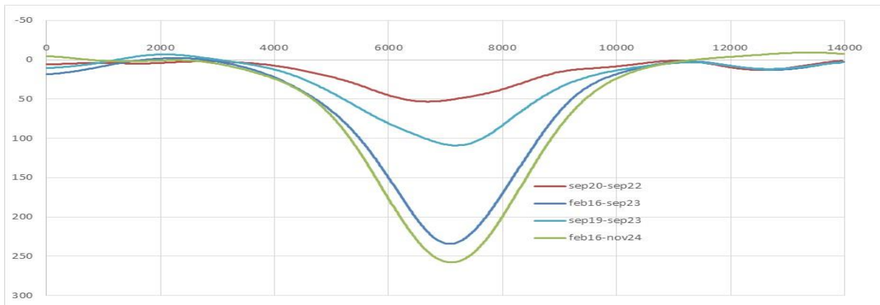
Figuur 4.6 : Insar bodemdaling W-E feb 2016 – nov 2024 en drie andere periodes.
