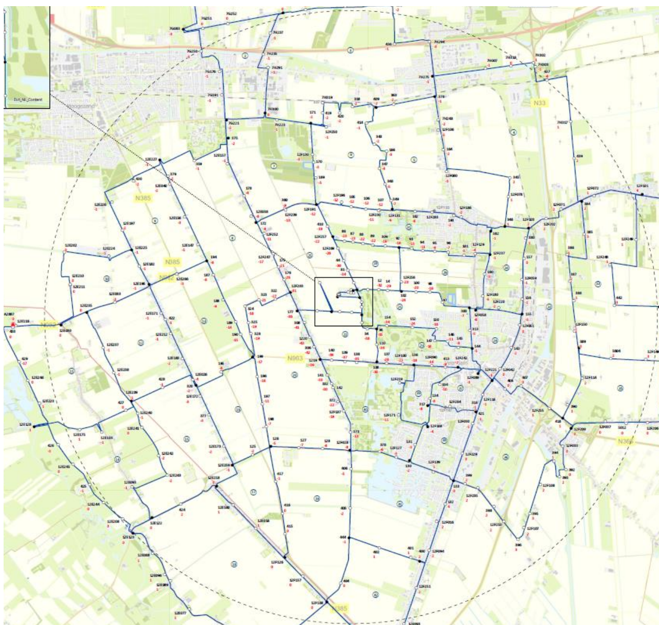
Figuur 4.4a: Waterpasmeetnet Nedmag in 2024, deels overlappend met het NAM meetnet met dalingen (indien negatief) in mm tussen 2022 en 2024.
