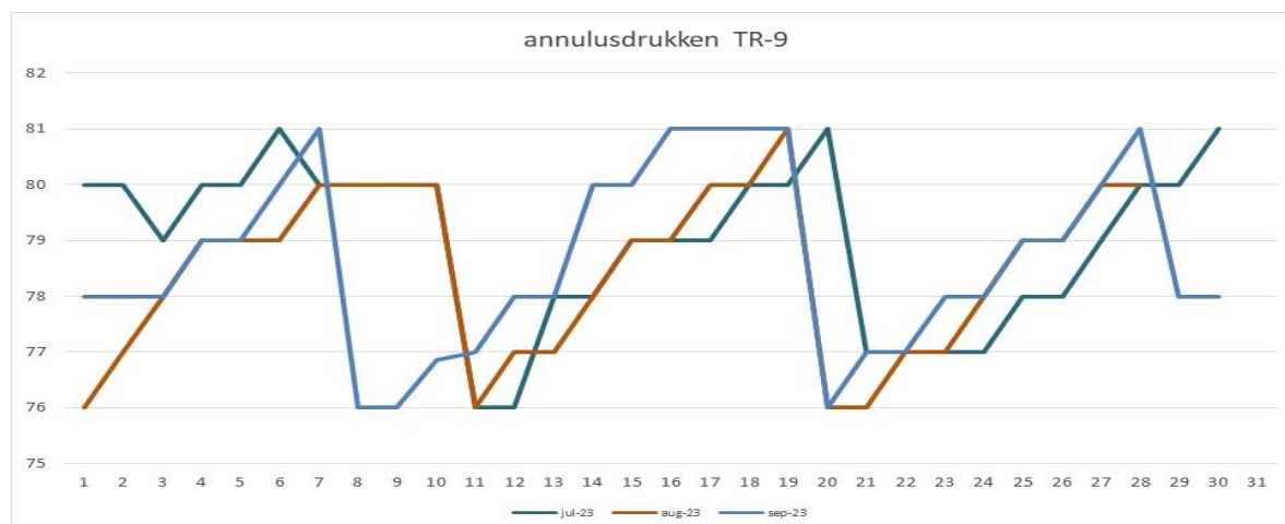
Figuur 1.5 drukverloop annulusdruk van TR-9 in Q3-2023.
