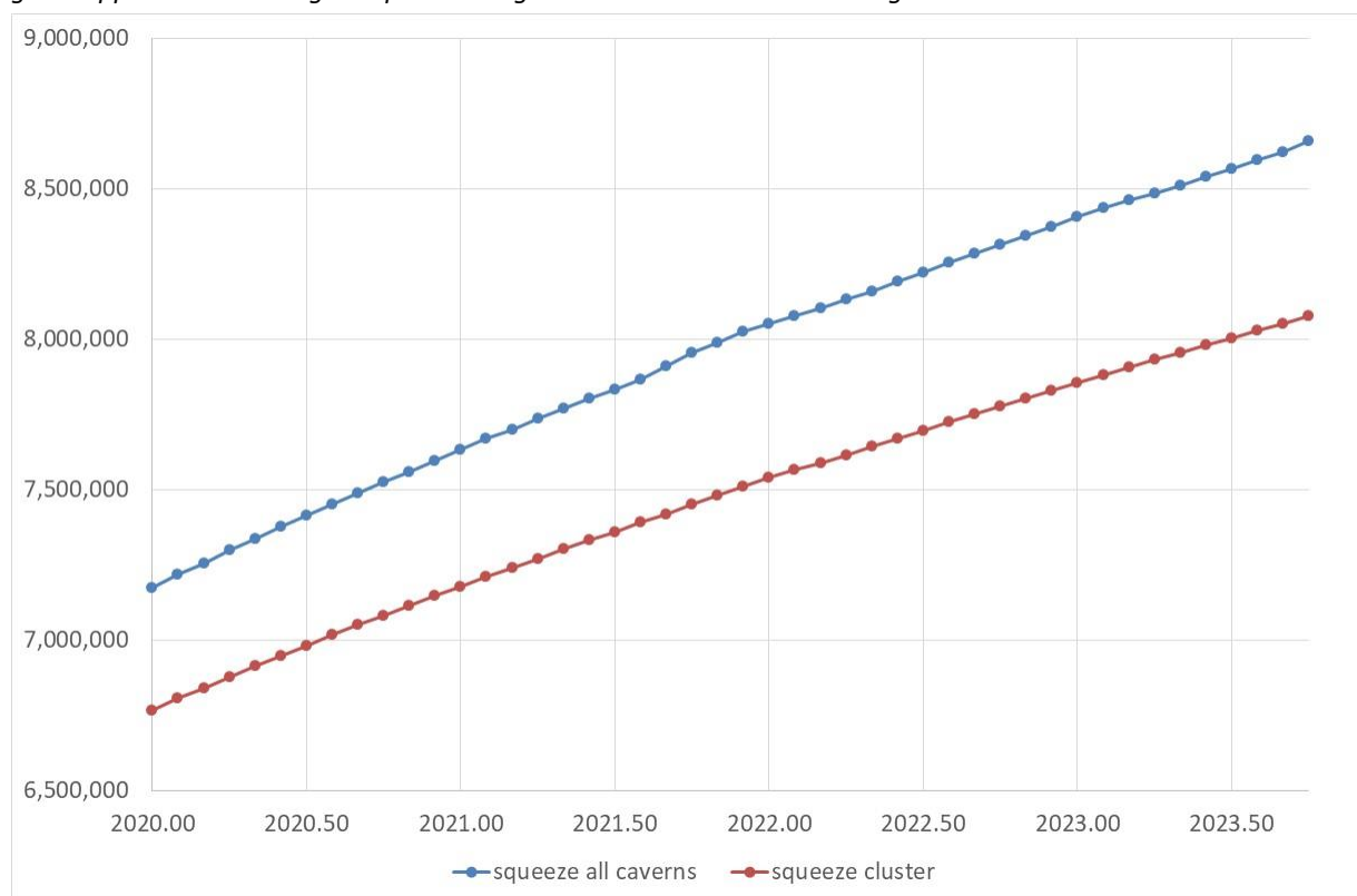
Figuur 4.1: cumulatieve squeeze-evolutie (caverneconvergentie) in m 3 van jan-2020 t/m sep-2023.
