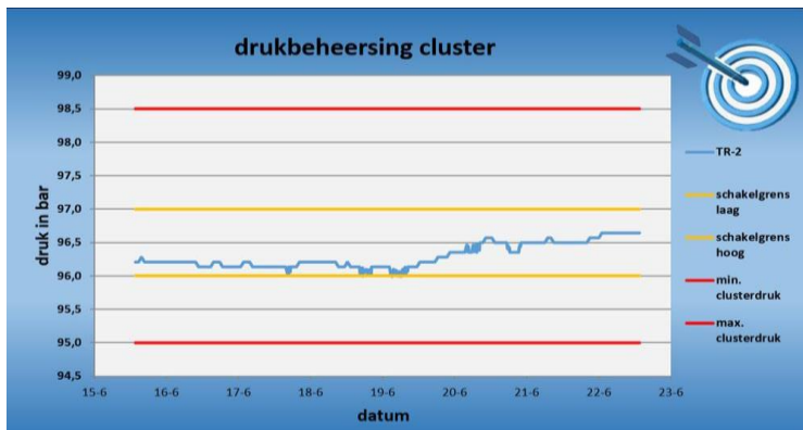
Figuur 1.1 Screenshot (juni 2023) van de maximum drukken cluster, basis TR-2
