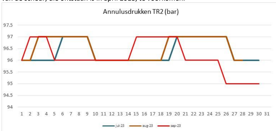
Figuur 1.3 drukverloop TR-2 in Q3-2023 (drukken zijn afgerond op hele bars).
