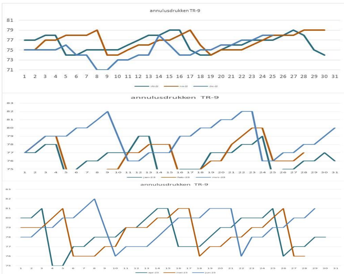
Figuur 1.6a/b/c. Drukverloop annulus TR-9 in Q4-22 t/m Q2-23.
