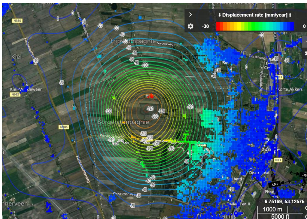
Figuur 4.3 Bodemdalingcontouren Insar feb 2016 t/m sep 2023 in mm. De gekleurde punten geven de gemiddelde (dus niet de actuele) dalingssnelheid van meetpunten van 0 tot 30 mm per jaar over deze zelfde periode. De contouren hebben hun eigen kleurenschaal van 0 tot 240 mm.
