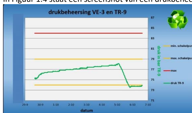
Figuur 1.4 drukverloop TR-9 als verloop van tijd, met als rode lijn de alarm druk (0-2 bar beneden maximum) aan het wellhead, afgeleid van de maximum casingschoendruk. De gele lijnen zijn gewenste operating-drukken bij normaal bedrijf.
