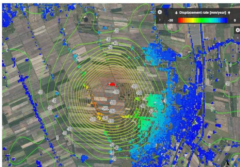
Figuur 4.3 Bodemdalingcontouren Insar feb 2016 t/m november 2022 in mm. De gekleurde punten geven de gemiddelde dalingssnelheid van meetpunten van 0 tot 30 mm per jaar over deze zelfde periode.
