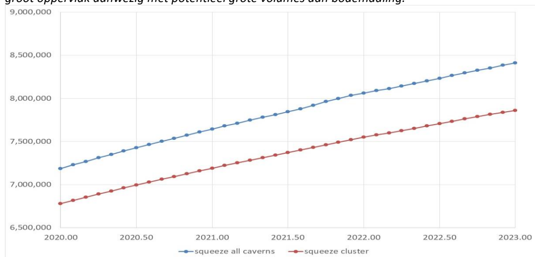
Figuur 4.1: cumulatieve squeeze-evolutie (caverneconvergentie) in m^3 van jan-2020 t/m dec-2022.
