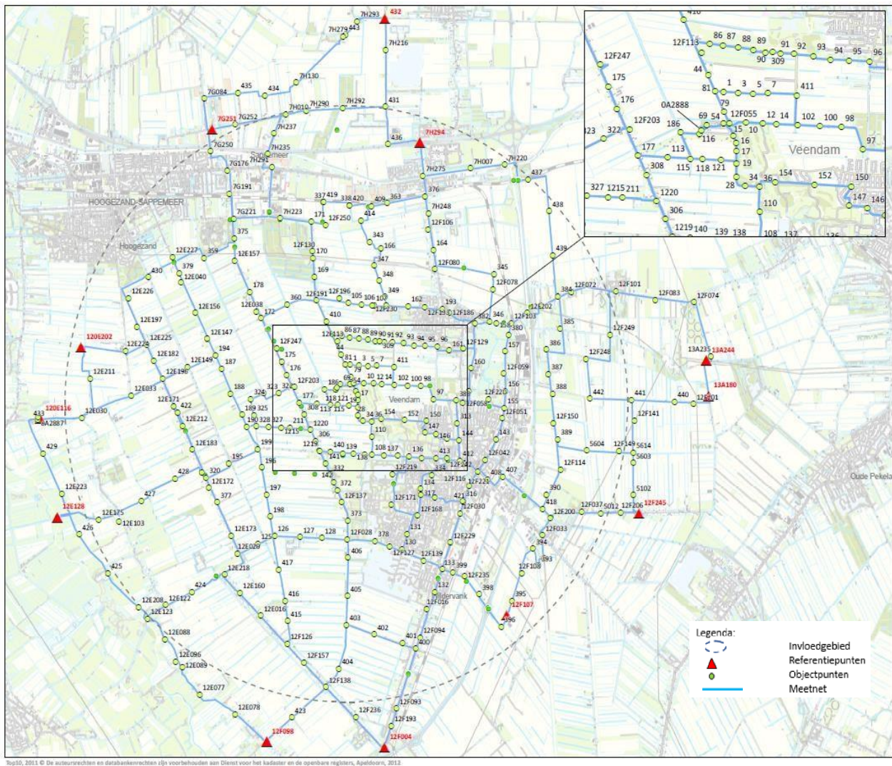
Figuur 4.4: Waterpasmeetnet Nedmag in 2018 en 2020, deels overlappend met het NAM meetnet.
