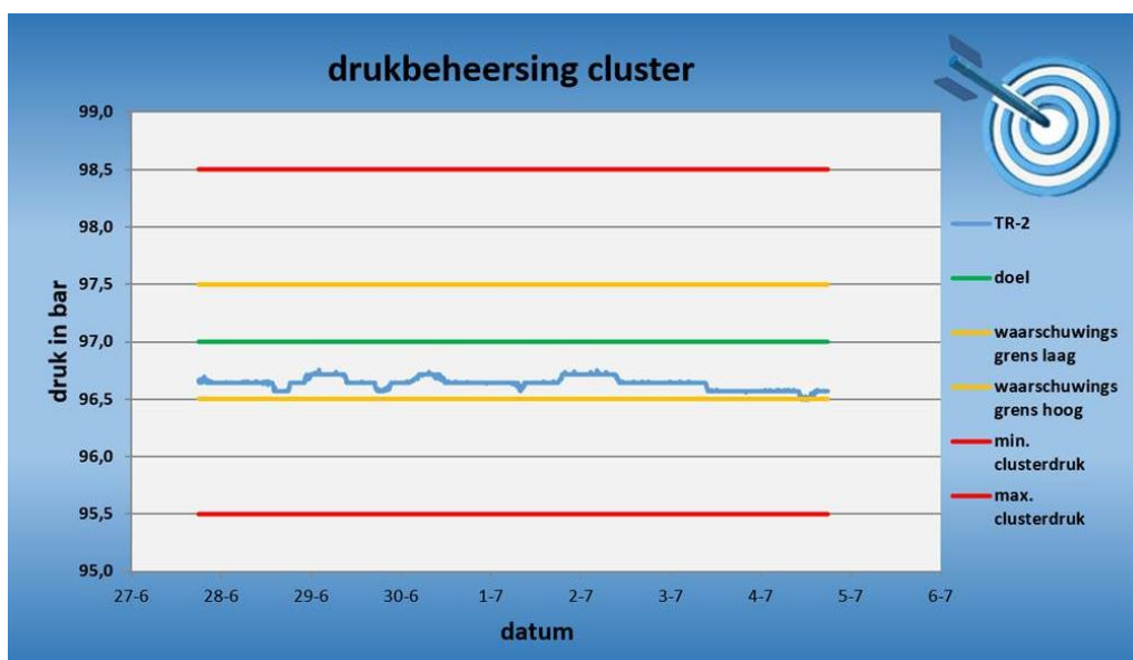
Figuur 1.1 Screenshot (juli 2022) van drukken en maximum drukken cluster, basis TR-2
