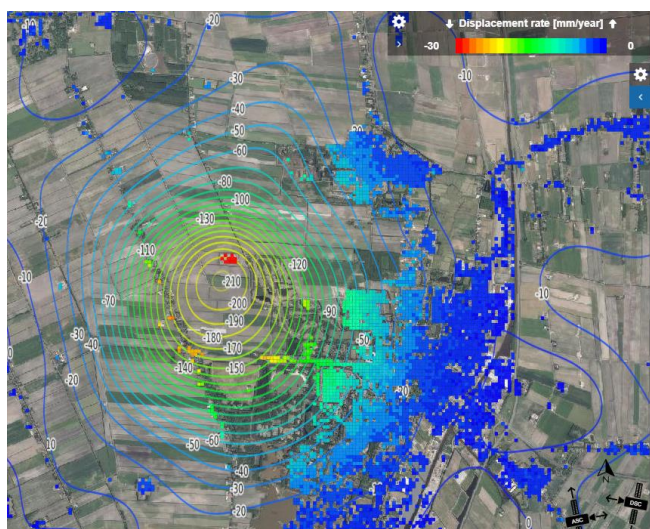
Figuur 4.3 Bodemdalingcontouren Insar feb 2016 t/m juni 2022 in mm. De gekleurde punten geven de gemiddelde dalingssnelheid van meetpunten van 0 tot 30 mm per jaar over deze zelfde periode.
