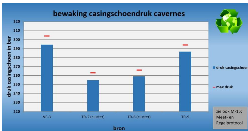
Figuur 1.2 Screenshot (juli 2022) van drukken en maximum drukken op casingschoenniveau voor het cluster (putten TR-2 en back-up meting TR-6) en voor de cavernes VE-3 en TR-9.
