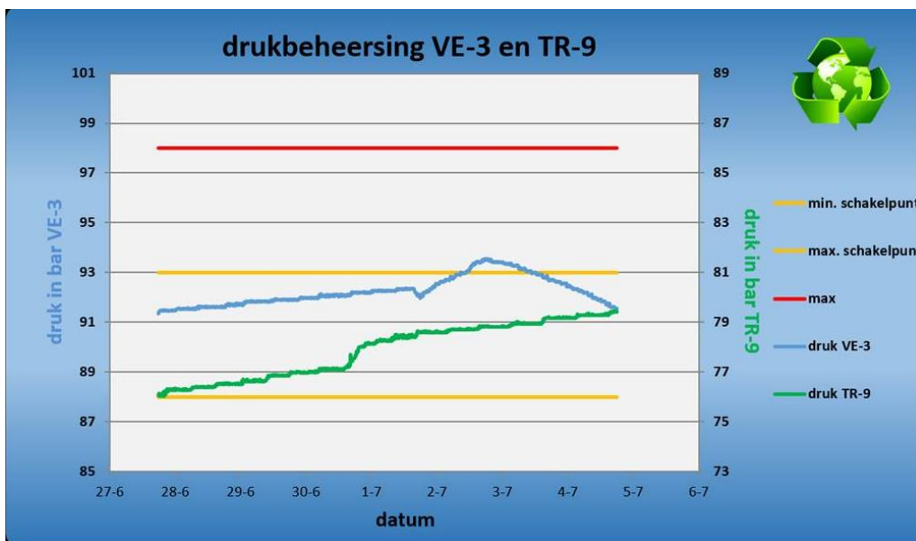
Figuur 1.4 drukverloop VE-3 (linkeras) en TR-9 (rechteras) als verloop van tijd, met als rode lijn de alarm druk (0-2 bar beneden maximum) voor beide putten aan het wellhead, afgeleid van de maximum casingschoendruk. De gele lijnen zijn gewenste operating-drukken bij normaal bedrijf van de fabriek aan de Billitonweg.
