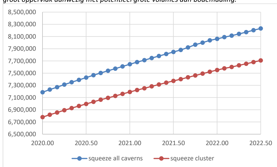
Figuur 4.1: squeeze-evolutie (caverneconvergentie) in m^3 van 2020 t/m Q2-2022.
