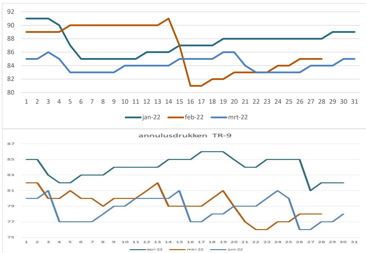
Figuur 1.6a/b. Drukverloop annulus TR-9 in Q1 en Q2-2022.
