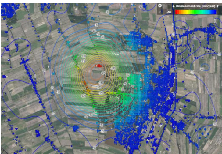
Figuur 4.3 Bodemdalingcontouren Insar feb 2016 t/m maart 2022 in mm. De gekleurde punten geven de gemiddelde dalingssnelheid van meetpunten van 0 tot 30 mm per jaar over deze zelfde periode.
