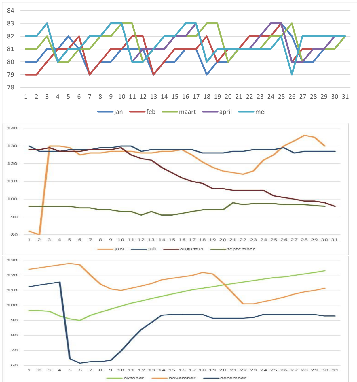
Figuur 1.5-a/b/c drukverloop annulusdruk van TR-9 in voorgaand jaar (2021). Begin juni is de annulusvloeistof vervangen van pek (1.30 kg/l) naar water, wat een drukstijging aangeeft. Vanaf augustus is de cavedruk verlaagd voorafgaand aan de workover. Per 5 december zit er weer pek (1.3 kg/l) in annulus.
