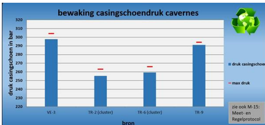
Figuur 1.2 Screenshot (feb 2022) van drukken en maximum drukken op casingschoenniveau voor het cluster (putten TR-2 en back-up meting TR-6) en voor de cavernes VE-3 en TR-9.
