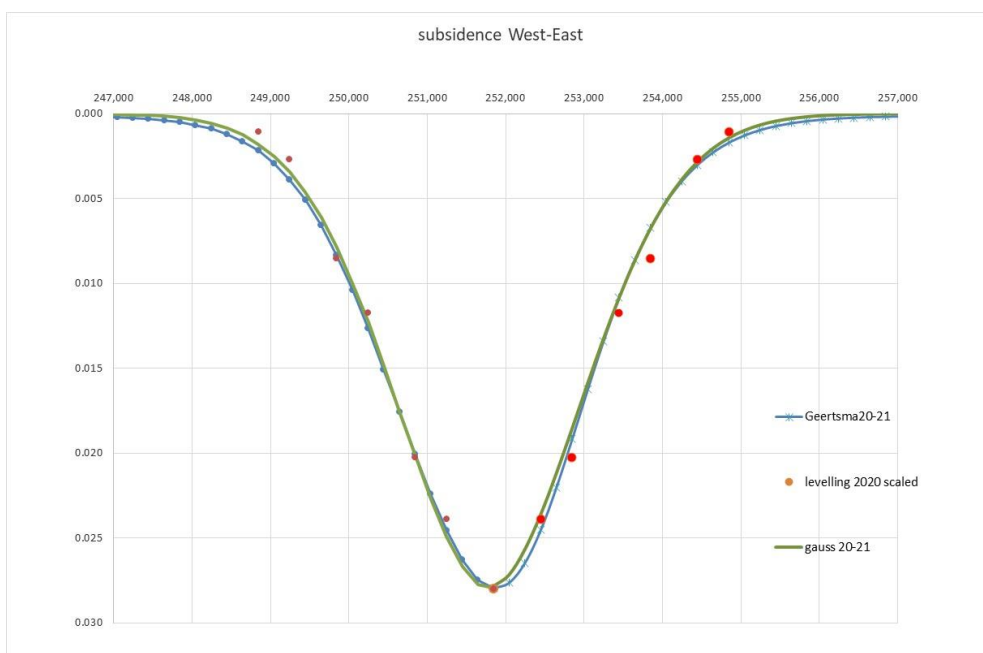
Figuur 4.7 : fit west-oost bodemdaling sep20-sep-21 volgens Geertsma (SGS-model) en Gauss curve met geschaalde waterpas (levelling) data 1993-2020, als functie breedte-coordinaten (Easting). Northing is 571 088 m
