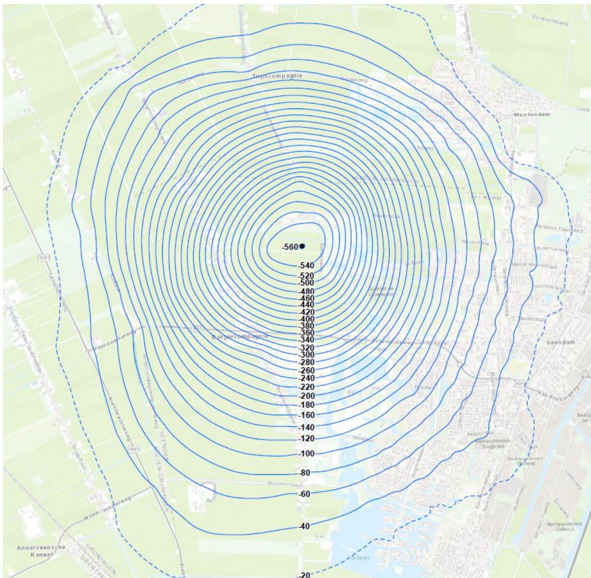
Figuur 4.5: Waterpasmeetresultaten Nedmag 1993- juni 2020 aangevuld met Insar daling juni 2020-augustus 2021
