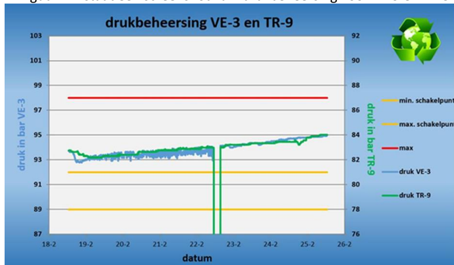
Figuur 1.4 drukverloop VE-3 (linkeras) en TR-9 (rechteras) als verloop van tijd, met als rode lijn de alarm druk (1 of meer bar beneden maximum) voor beide putten aan het wellhead, afgeleid van de maximum casingschoendruk. De gele lijnen zijn de grenzen van de gewenste operating-drukken bij normaal bedrijf van de fabriek aan de Billitonweg. Bij een serverstoring of reboot (zie 22-2) kunnen kortstondig waardes wegvallen.
