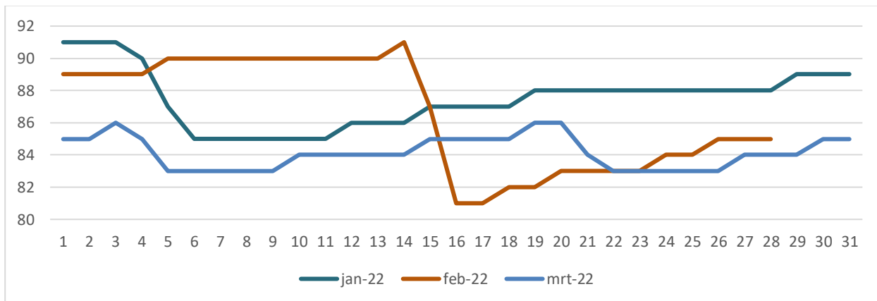
Figuur 1.6. Drukverloop annulus TR-9 in Q1-2022.
