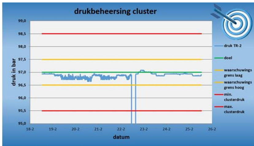
Figuur 1.1 Screenshot (feb 2022) van drukken en maximum drukken cluster, basis TR-2
