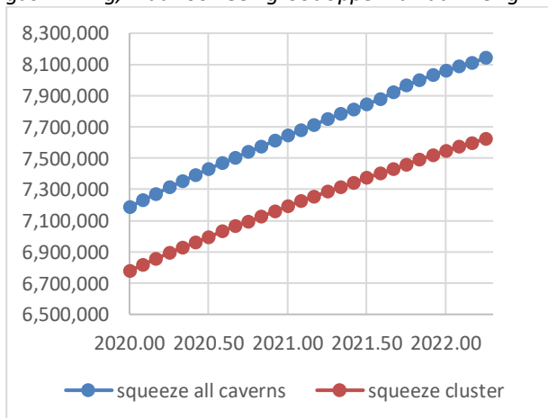
Figuur 4.1: squeeze-evolutie (caverneconvergentie) in m^3 van 2020 t/m Q1-2022.
