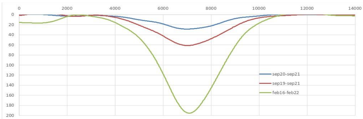
Figuur 4.6 : Insar bodemdaling feb 2016 – feb 2022 en recente dalingen over 1 en 2 jaar.
