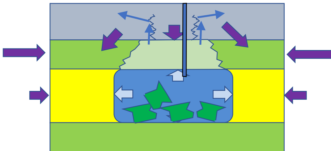
Figuur 15: Instorten van een (halietaak) zoutdak doordat de schuifspanningen in het dak te hoog worden. Er ontstaat directe verbinding tussen de caverne en het bovenliggende doorlatende Buntzandsteen. De paarse pijlen geven gesteentespanningen aan, de lichtblauwe pijlen vloeistofdrukken en de blauwe dunne pijlen de stroming van de vloeistof.
