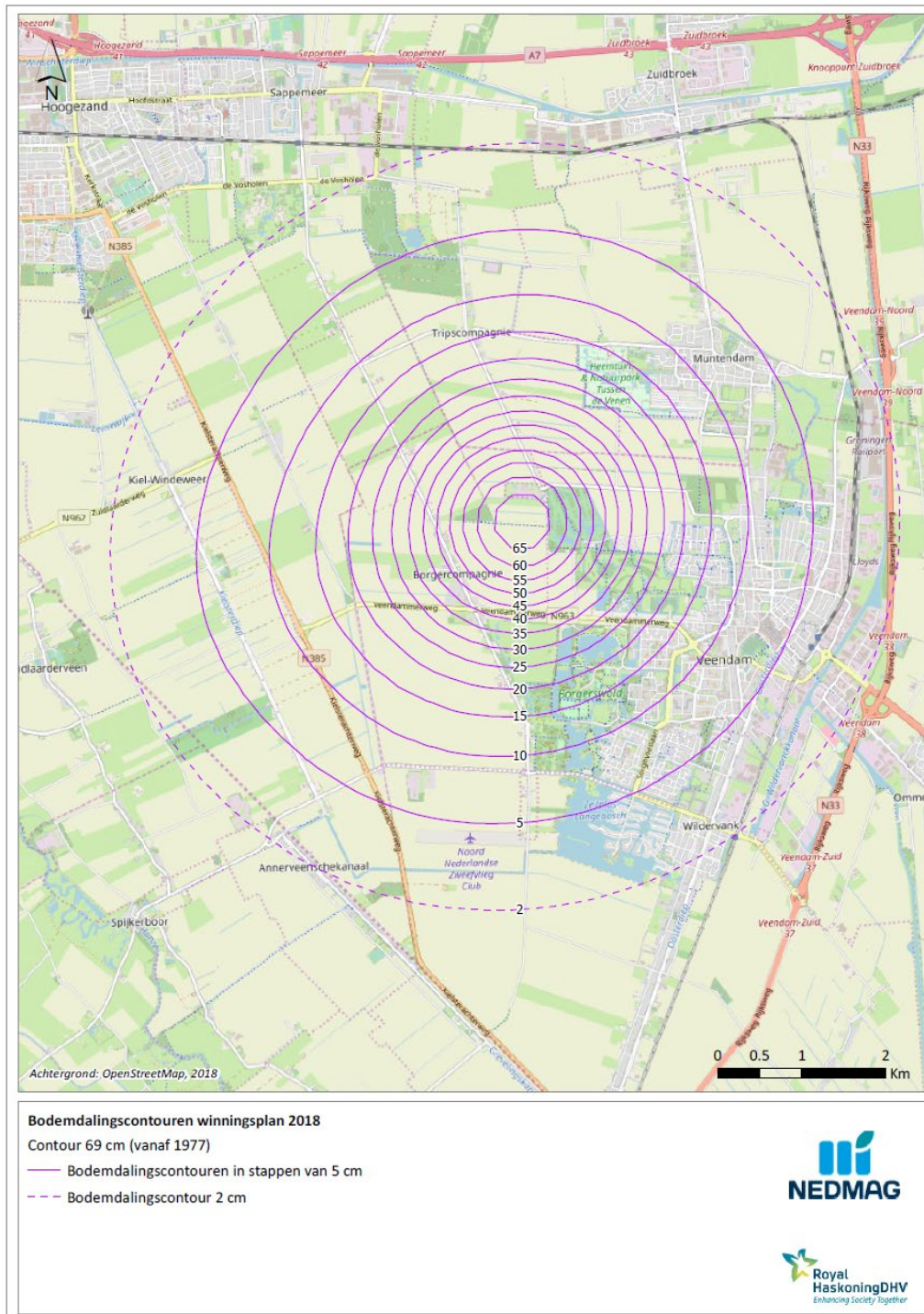
Figuur 24: Bodemdalingscontour vanaf 1977 na afdalen vrije pekkel uit TR-cluster en na actieve winning uit bronnen TR-9, VE-3 en VE-5 tot en met VE-8.
