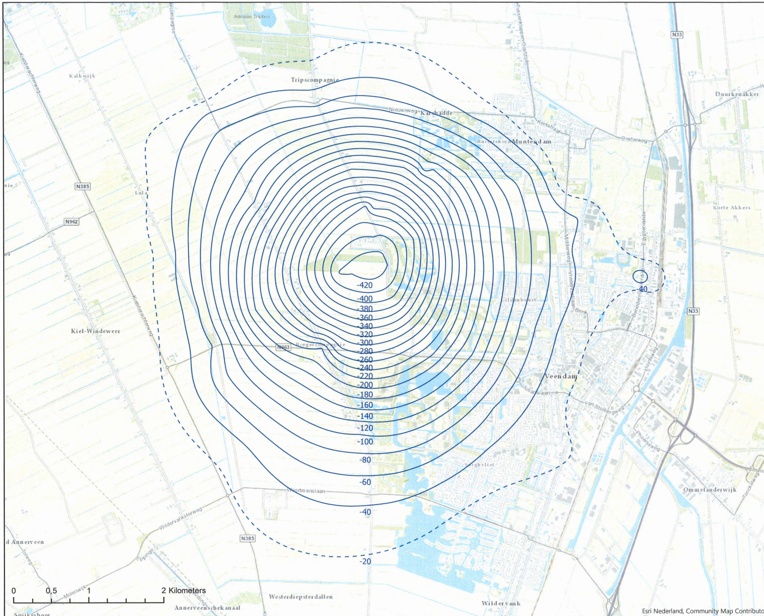
Deze kaart geeft de bodemdaling door zoutwinning over de periode 1993 - 2018 aan. De bodemdaling vóór 1993 was ca. 4 cm in het centrum.
